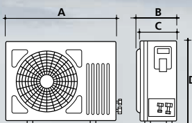
Unità esterna SOS 30
