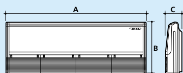
Unità interna SSU 44-52
