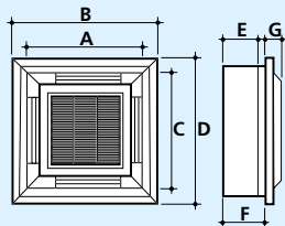
Unità interna SSC 17-24-30
