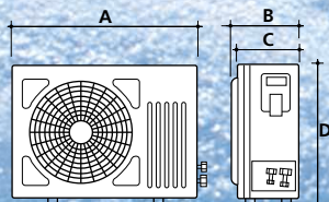
Unità esterna SOS 24-30 / SOR 24
