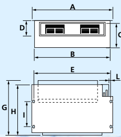
Unità interna SPD
