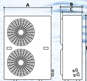
Unità esterna SOS 44-52-60
